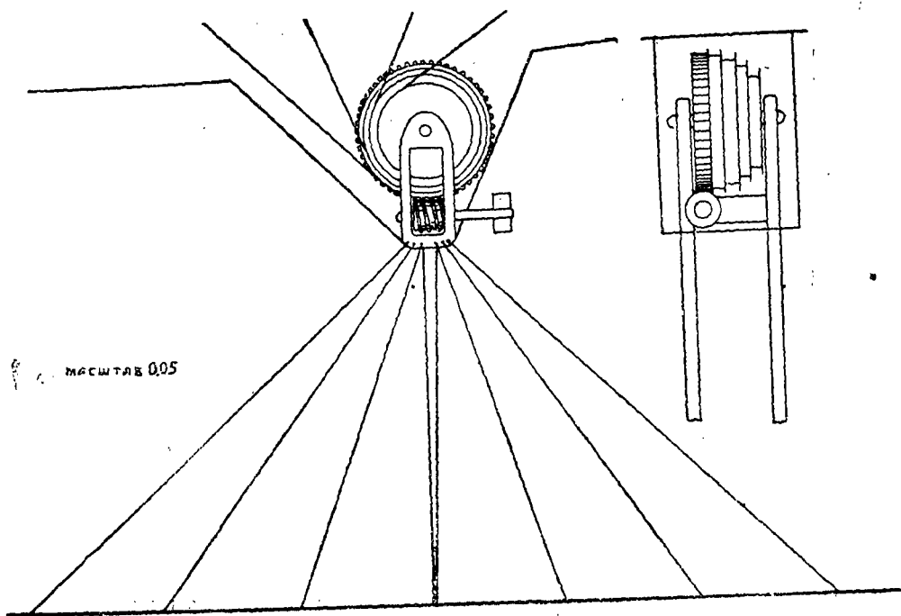
Черт. 13. 0,02 = 1:50 .
