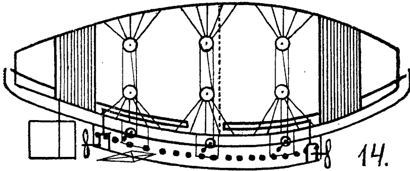
14. Схема металлического дирижабля. Верхнее основание. Блочное стягивание. Черные трубы для нагревания газа. Нижнее основание с прилегающими к нему камерами с валами для наматывания тросов блочной системы. Гондола. Рули. Моторы с гребными винтами. Ряд окон.
