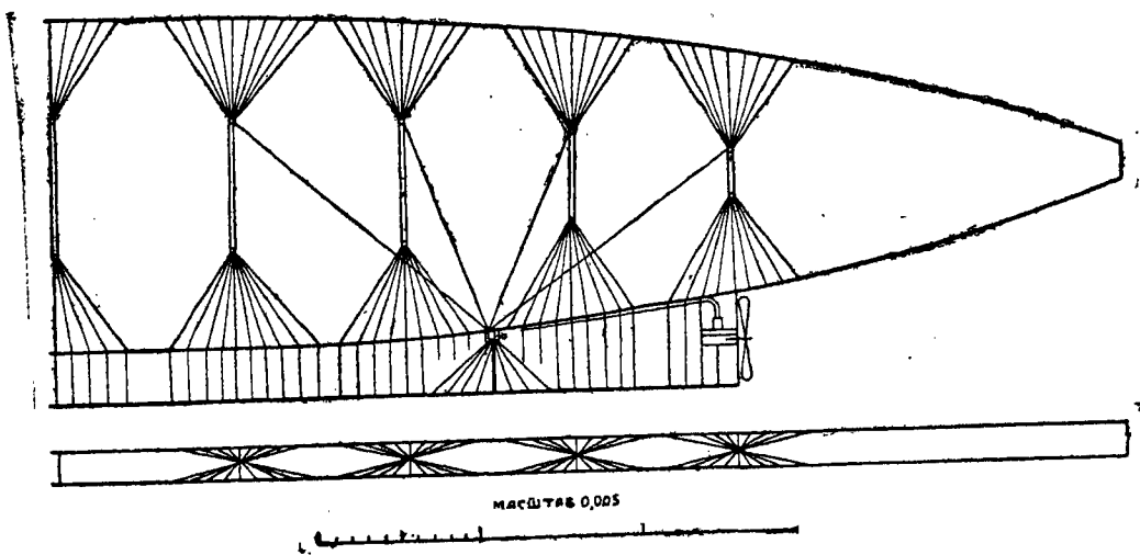
Черт. 4. 1:500.
