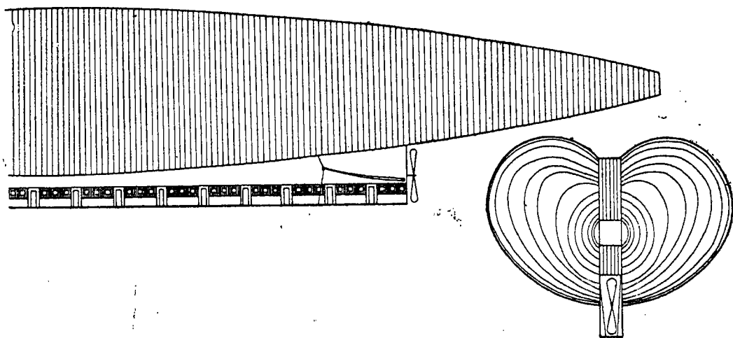
Черт. 6. 1:500.
