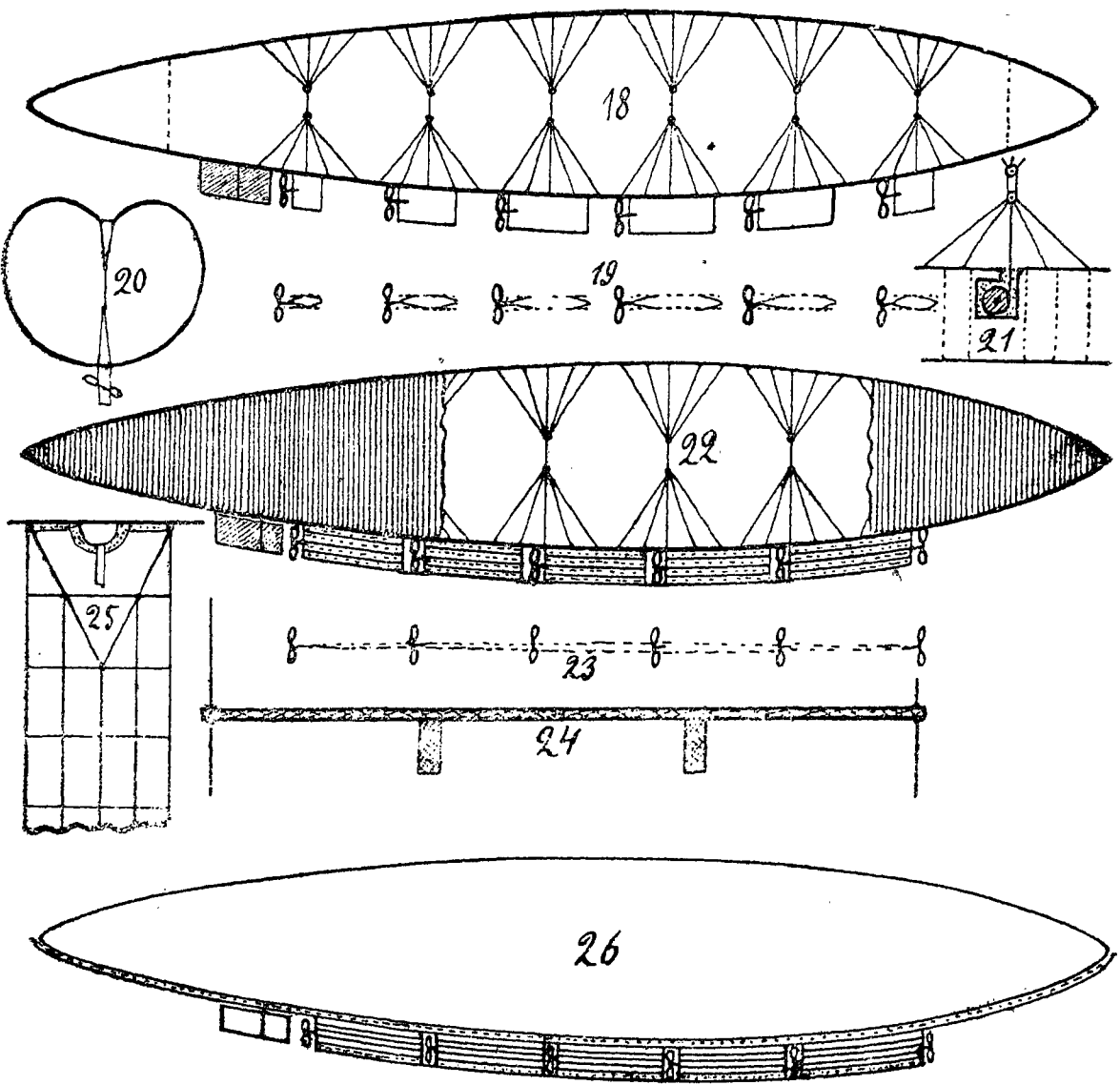
18—26. Старые проекты. 20. Поперечное сечение. 21. Камера со стягивающим валом. 24. Пол гондолы. 25. Поперечное сечение многостажной гондолы. Сверху — нагревающая труба.
