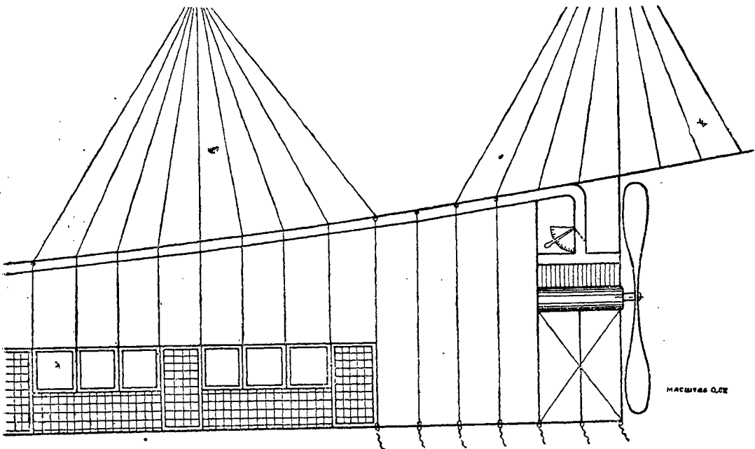
Черт. 15. 0,008 = 1 : 125.
