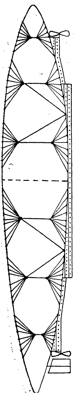
27. Продольное отгвесное сечение дрижабля на 200 человек. Пропорциональный чертеж.
